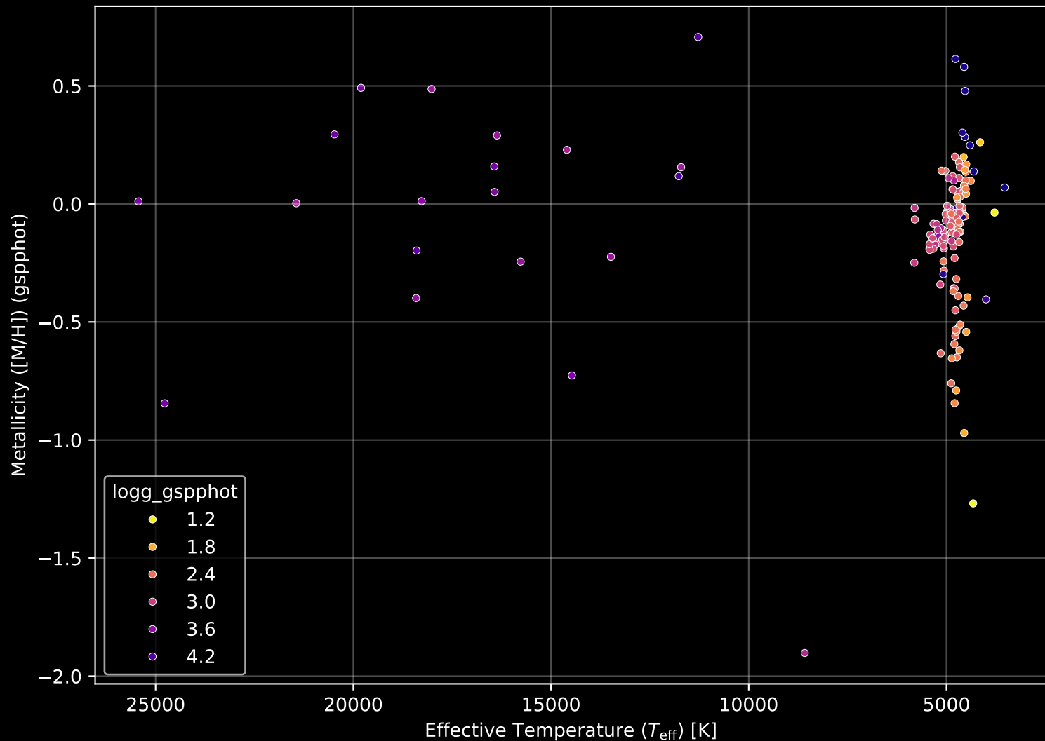
APOGEE DR17 Field: [135-06] Stellar Population Parameters (n= 156)
